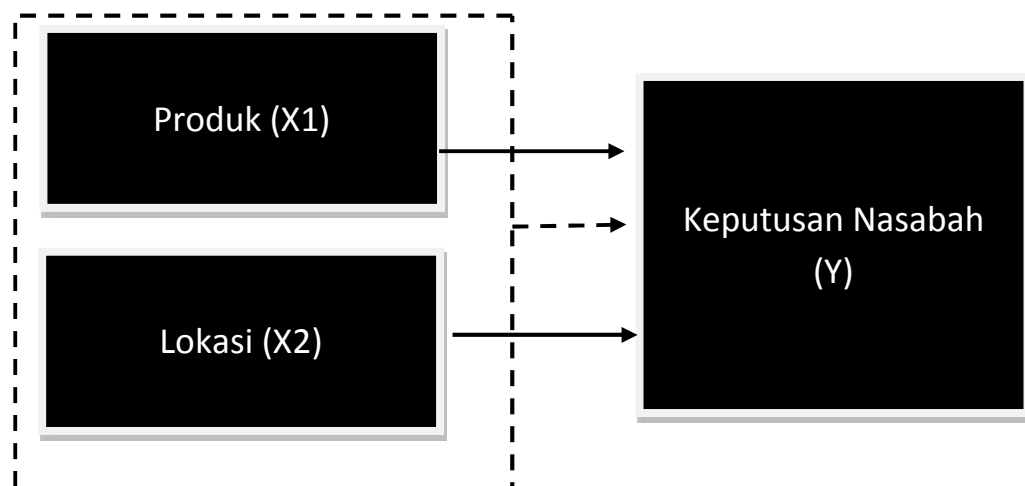
Gambar 1 Kerangka Pemikiran
