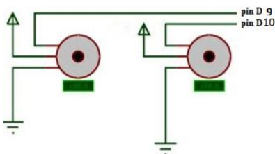
Gambar 12. Rangkaian Motor Servo
