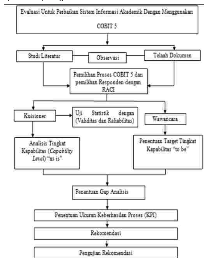
Gambar 1. Metodologi Penelitian
