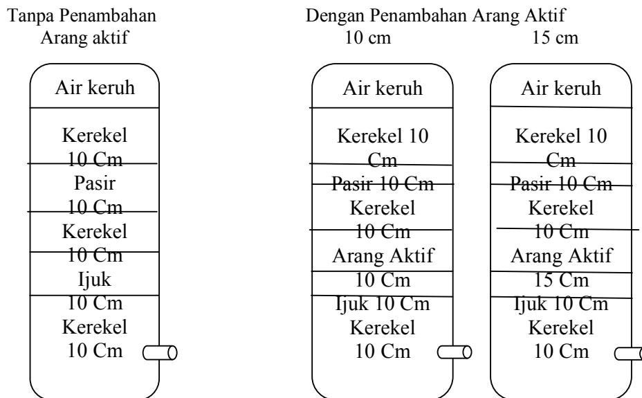
Gambar 1 : Saringan pasir lambat pada proses filtrasi air sumur
