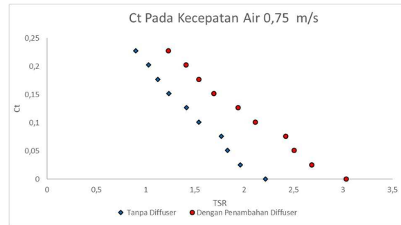
Gambar 15. Grafik Torque Coefficient Terhadap TSR pada v = 0,75 m/s
