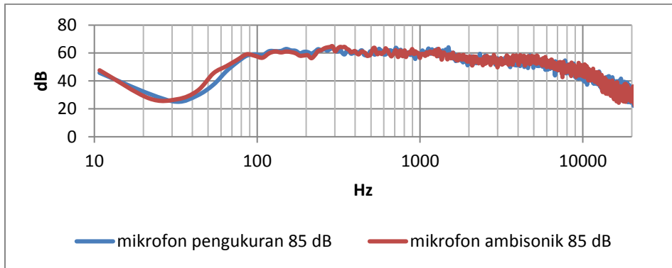
Gambar 8 Respon Frekuensi Mikrofon Pengukuran dan Mikrofon Ambisonik pada 85 dB
