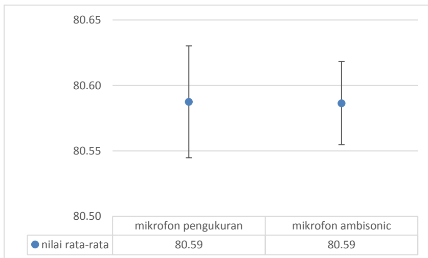
Gambar 9 Hasil Pengukuran pada sinyal “White Noise” pada 80 dB
