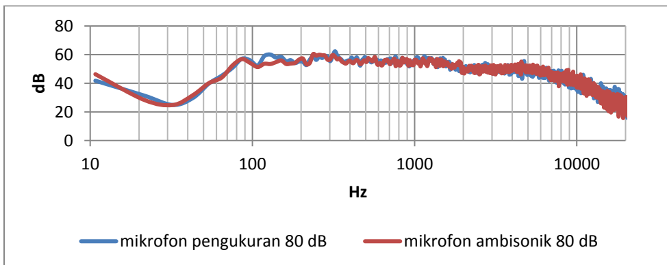
Gambar 7 Respon Frekuensi Mikrofon Pengukuran dan Mikrofon Ambisonik pada 80 Db
