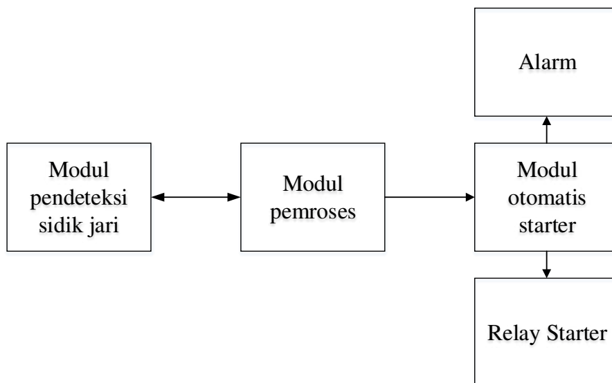
■ Gambar 3. Diagram Blok Keseluruhan Sistem
