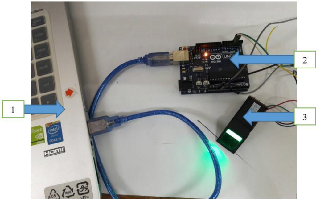
■ Gambar 6. Tampilan Fisik Modul Registrasi
