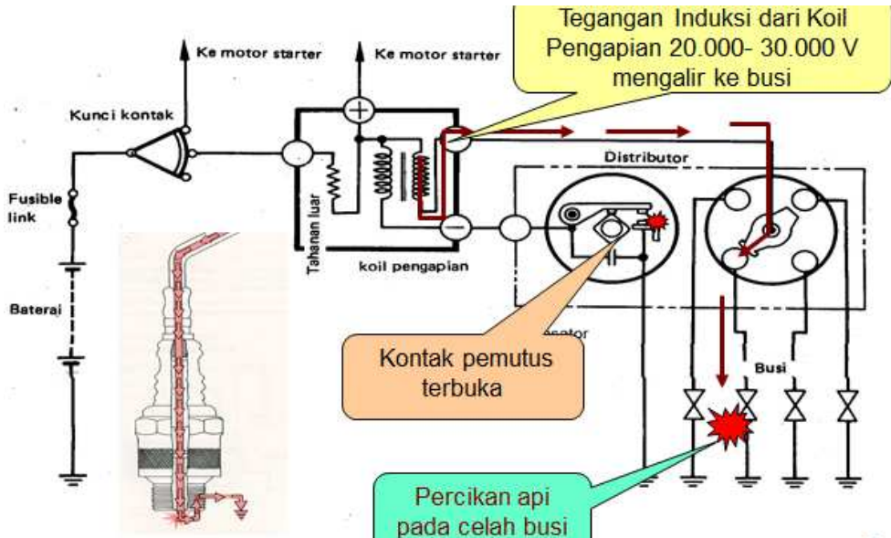
■ Gambar 8. Schematic Sistem Kelistrikan Pada Kontak Mobil
