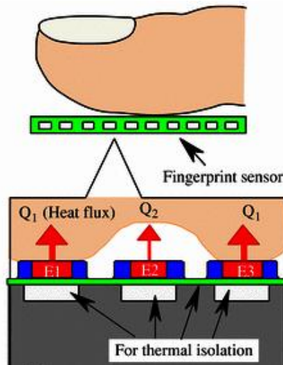
■ Gambar 5. A. Pembacaan Sidik Jari Secara Optis B. Pembacaan Sidik Jari Secara kapasitan C. Pembacaan Sidik Jari Secara Thermal
