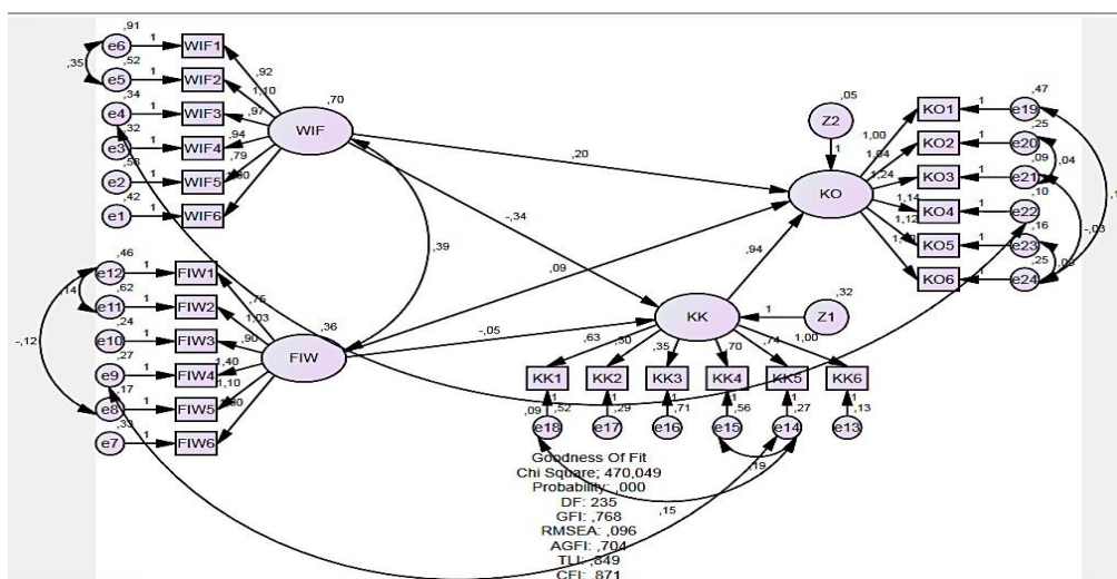
GAMBAR 1 Model Pengukuran
