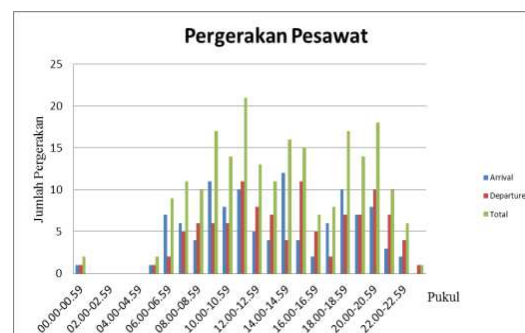
Gambar 1 Jumlah Setiap Tipe Pesawat pada 111 penerbangan turnaround
