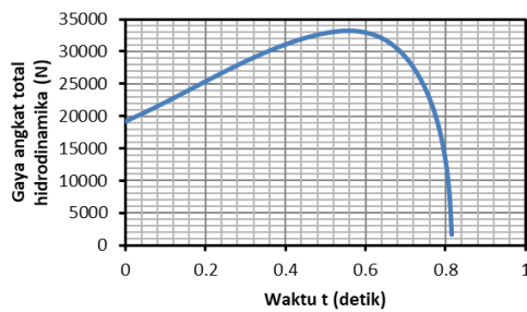
Gambar 5. Kurva gaya angkat total hidrodinamika L_{hidro} versus waktu t pada pergerakan pesawat WISE L8 berkapasitas 8 Orang fase take off.
