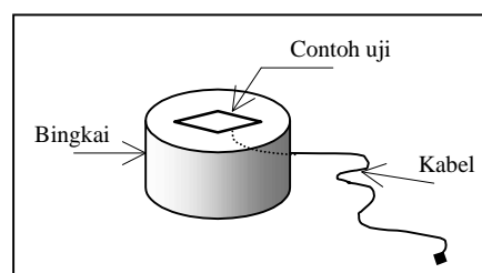
Gambar 2. Skematis contoh uji yang telah siap diuji korosi
