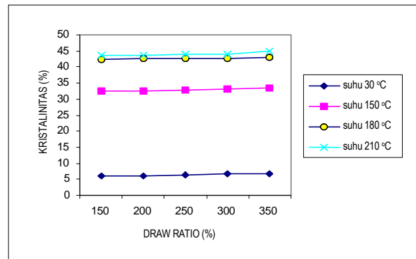
Gambar 1. Hubungan kristalinitas terhadap draw ratio dan suhu penarikan serat poliester.
