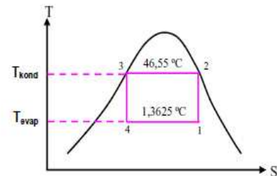
Gambar 4.3. Diagram T-S siklus Carnot
