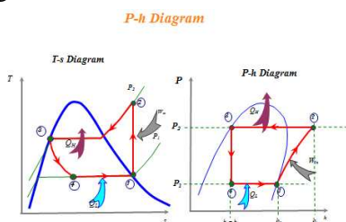
Gambar 3.7 Siklus kompresi uap
