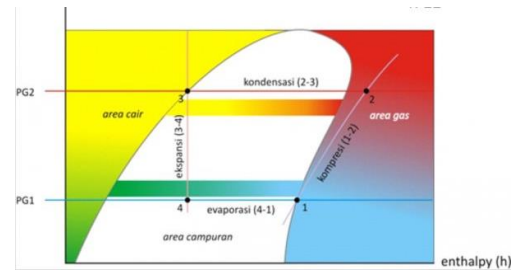
Gambar 3.8 Siklus perubahan fase
