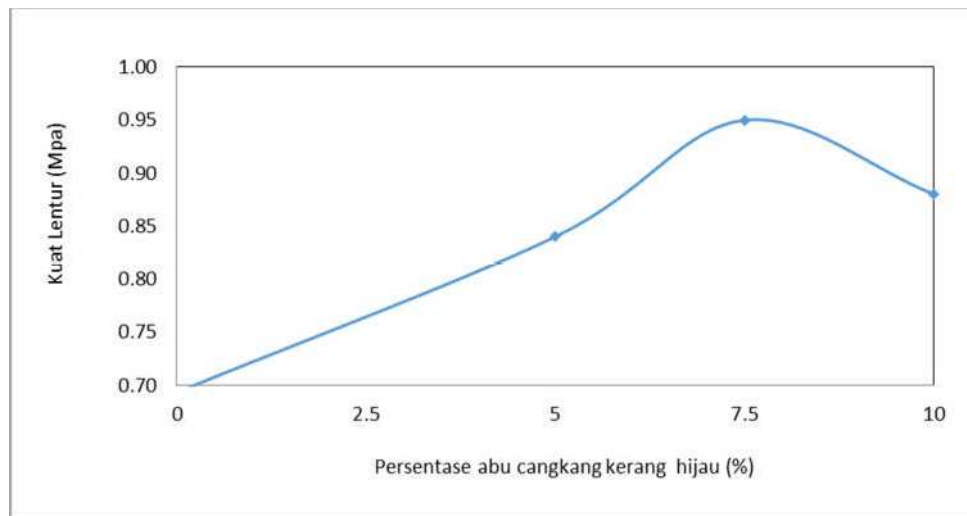
Gambar 3. Hubungan kuat lentur dengan persentase abu cangkang kerang hijau
