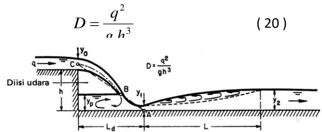
Gambar 3. Geometri aliran pada pelimpah terjunan lurus.
