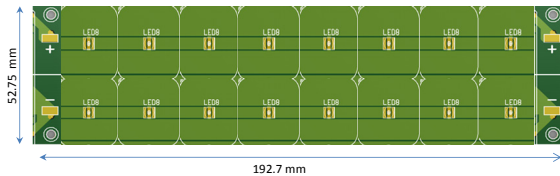
Gambar 11. PCB dengan material aluminium core untuk lampu 12 buah LED
