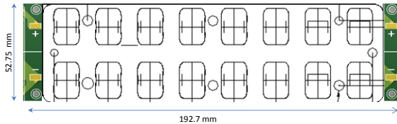
Gambar 12. PCB dan Lensa yang sudah di assembly untuk lampu 12 buah LED
