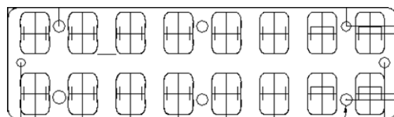
Gambar 10. Model Lensa untuk lampu 12 buah LED
