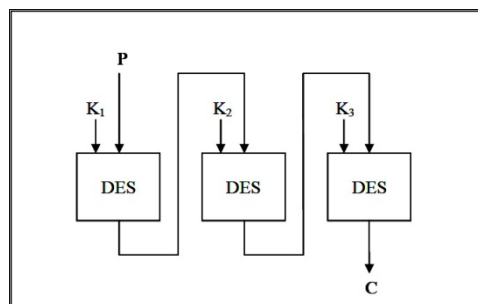
Gambar 2. Skema algoritma Triple DES
