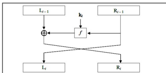
Gambar 1. Jaringan Feistel untuk satu putaran DES
