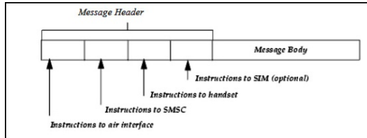
Gambar 3. Struktur pesan SMS
