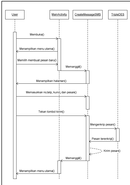
Gambar 9. Sequence Diagram membuat pesan baru
