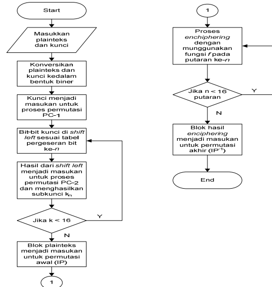
Gambar 5. Diagram alir algoritma DES
