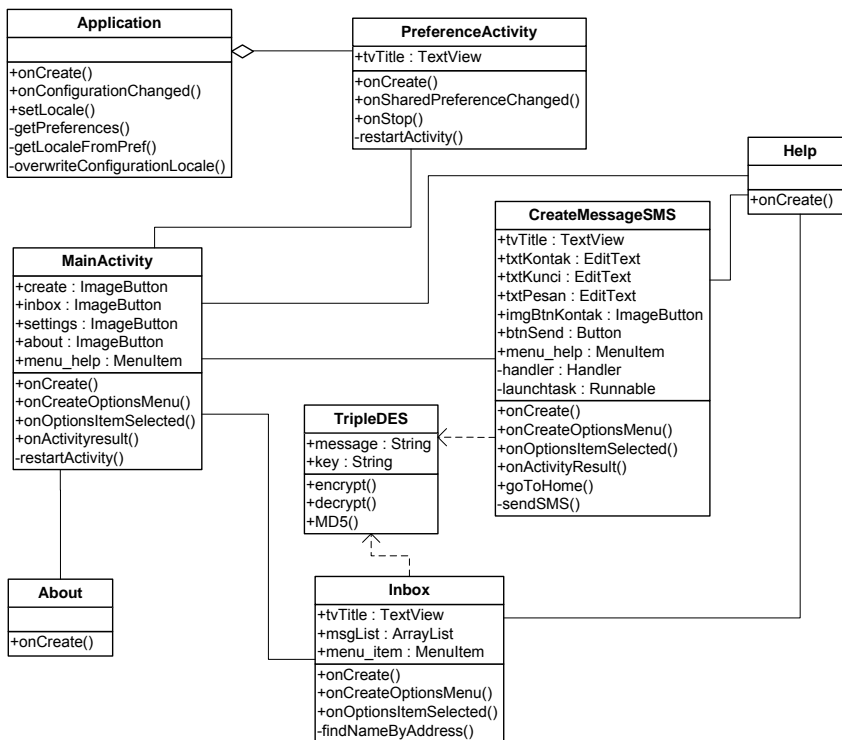
Gambar 8. Class diagram aplikasi Crypto Messenger
