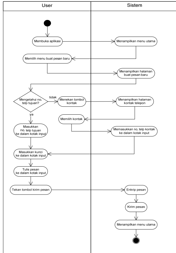
Gambar 7. Activity diagram membuat pesan baru
