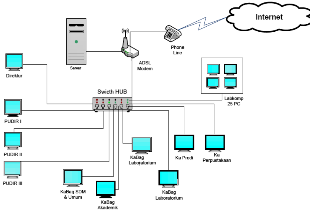
Gambar 3.2 Arsitektur SISFO-PIKSI
