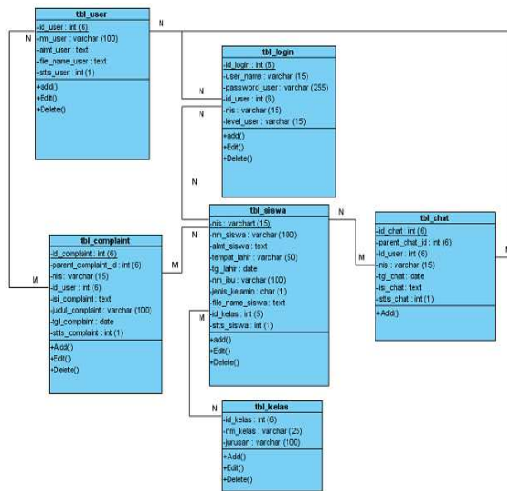
Gambar 3.4 Class Diagram Keluhan Siswa Yang Diusulkan
