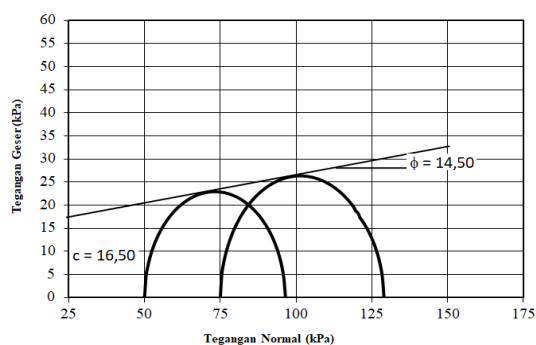
Gambar 6. Hasil Pengujian Triaksial Titik 2A
