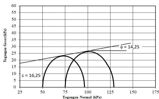
Gambar 7. Hasil Pengujian Triaksial Titik 2B
