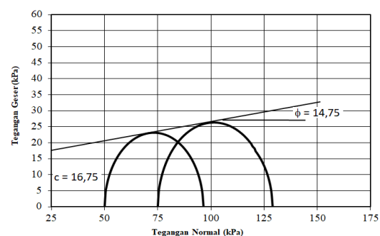
Gambar 8. Hasil Pengujian Triaksial Titik 3A
