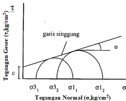
Gambar 2. Lingkaran Mohr Sumber :Das (1995)
