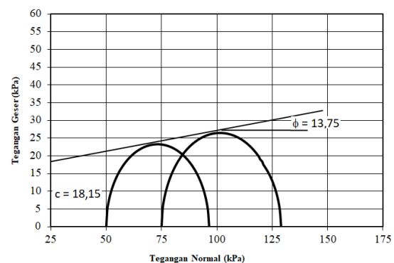
Gambar 5. Hasil Pengujian Triaksial Titik 1B
