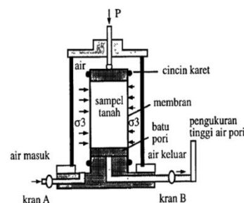
Gambar 1. Skema Pengujian Triaksial Sumber :Das (1995)
