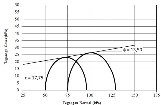
Gambar 4. Hasil Pengujian Triaksial Titik 1A
