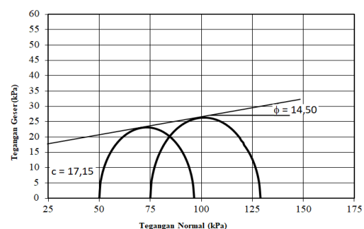
Gambar 9. Hasil Pengujian Triaksial Titik 3B
