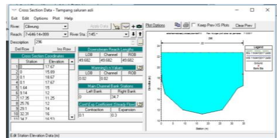
Gambar 4 Contoh Input Data Potongan Melintang
