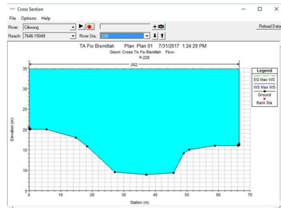
Gambar 9 Hasil Aliran Unsteady Debit Rencana 10 Tahun pada Potongan 228
