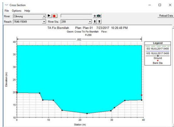
Gambar 6 Hasil Aliran Unsteady Debit Rencana 5 Tahun pada Potongan 299
