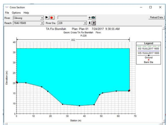
Gambar 11 Hasil Aliran Unsteady Debit Rencana 20 Tahun pada Potongan 228
