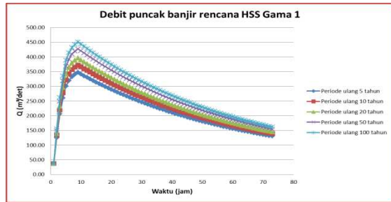
Gambar 2 Debit Puncak Banjir Rencana HSS Gama 1
