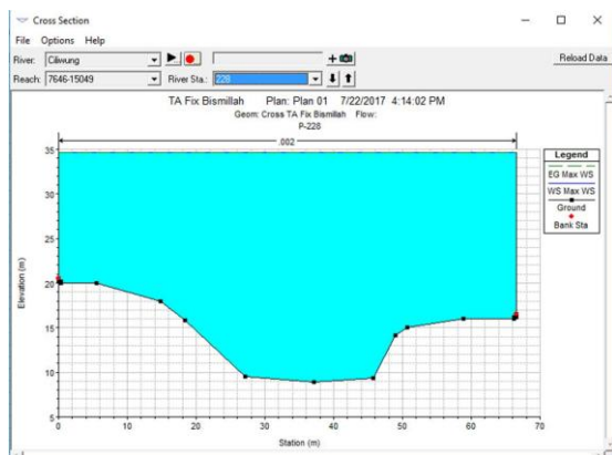
Gambar 7 Hasil Aliran Unsteady Debit Rencana 5 Tahun pada Potongan 228
