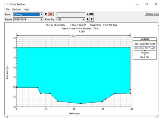
Gambar 8 Hasil Aliran Unsteady Debit Rencana 10 Tahun pada Potongan 299
