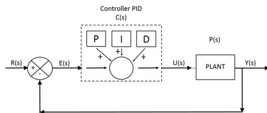
Gambar 3.1.a Kontrol PID
