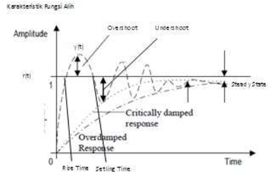
Gambar 3.1.b Kontrol PID
