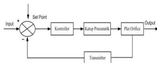
Gambar 2.3. Diagram Blok Sistem Pengontrolan
