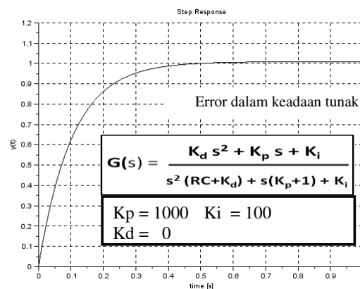
Gambar 4.3 Fungsi step yang terkait dengan aksi control P(s) dan PID
