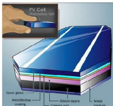
Gambar 2.1 Struktur Sel Surya
