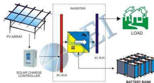
Gambar 2.7 Prinsip kerja PLTS-Terpusat
