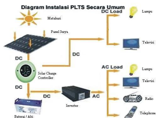
Gambar 2.2 Skema Instalasi PLTS
