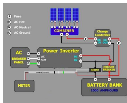
Diagram instalasi pembangkit listrik tenaga surya
