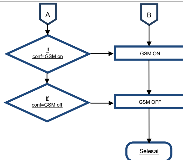
Gambar 2. Flowchart Alur Kerja Aplikasi
