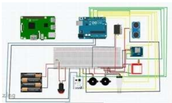
Gambar 3. Perancangan rangkaian
