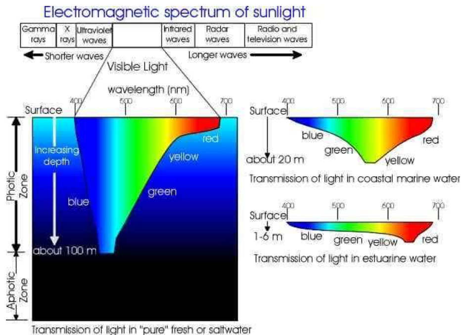
Gambar 13. Intensitas cahaya berwarna di dalam laut
