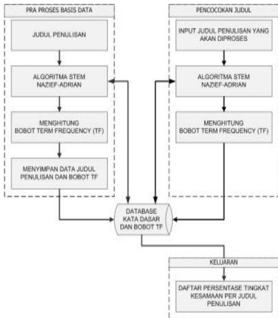
Gambar 1. Alur Pendeteksi Kesamaan Kata
