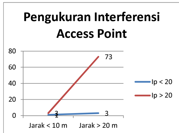
Gambar 7. Pengukuran Interferensi AP
