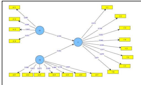
Gambar2.Hasil Pengujian Kelayakan SEM Convergent Validity
