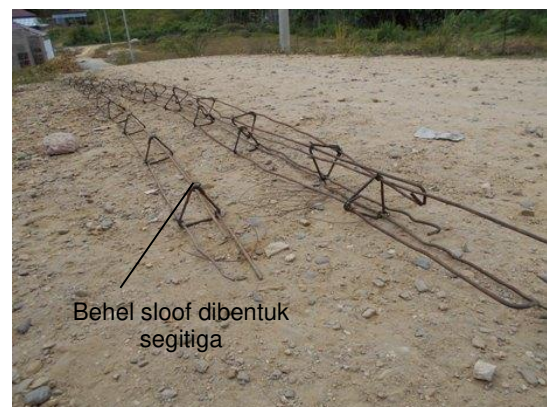
Gambar 4. Behel dibentuk segitiga pada sloof di Perumahan BTN di Kota Kendari Sumber : Hasil dokumentasi, 2017
