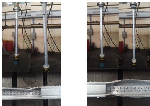
Gambar 7. Benda uji model 1 (kiri) dan model 2 (kanan) sebelum ditekan, saat ditekan, dan kegagalan yang terjadi
