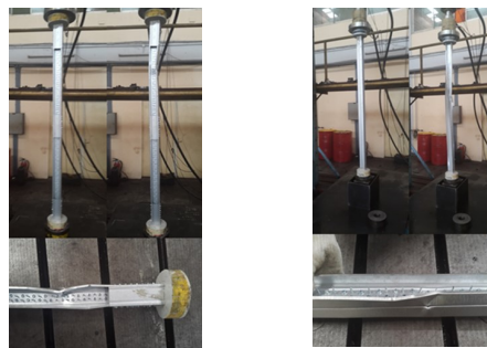
Gambar 8. Benda uji model 1 (kiri) dan model 2 (kanan) sebelum ditekan, saat ditekan, dan kegagalan yang terjadi
