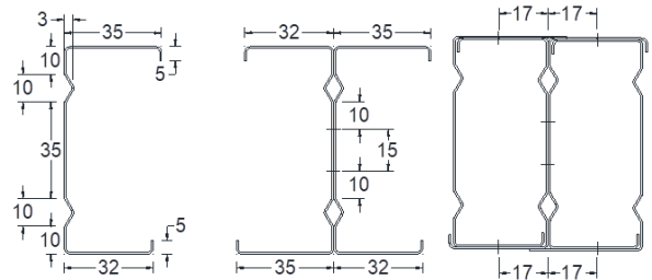
Gambar 4. Sketsa penampang kanal (kiri), penampang tersusun (tengah), dan penampang berpengaku (kanan)
