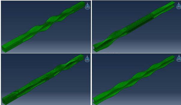
Gambar 9. Ragam tekuk hasil analisis elemen hingga model 1 (kiri atas), model 2 (kanan atas), model 3 (kiri bawah), dan model 4 (kanan bawah)
