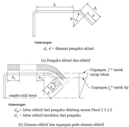
Gambar 2. Elemen dengan pengaku tepi lip sederhana (SNI 7971:2013)
