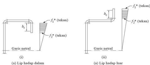
Gambar 1. Elemen tanpa pengaku dengan tegangan bergradien tekan (SNI 7971:2013)
