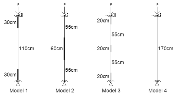
Gambar 5. Sketsa penempatan pengaku struktur benda uji
