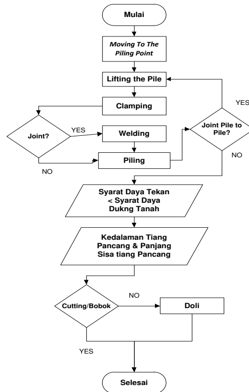
Gambar 5. Bagan alir proses 1 titik pemancangan
