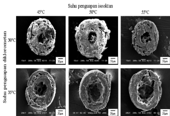
Gambar 5. Foto SEM mikrokapsul polistiren dengan berbagai variasi suhu penguapan.
