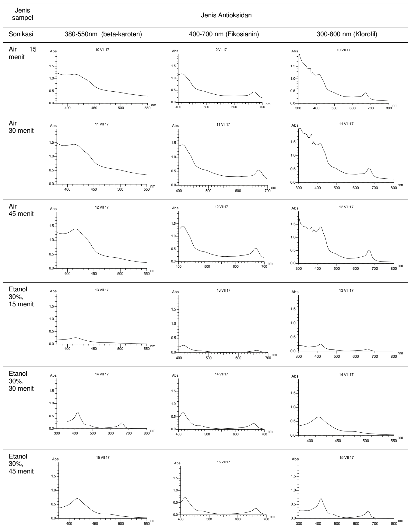
Gambar 2. Identifikasi jenis antioksidan dengan menggunakan spektrofotometer
