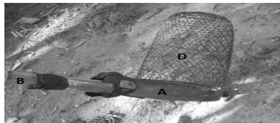
Gambar 2. Alat tangkap tangge yang digunakan dalam pengambilan sampel kerang pokea. Keterangan: (A = besi pelingkar, B = bambu, C = tali dan D = mata tangge) dalam berbagai ukuran.
