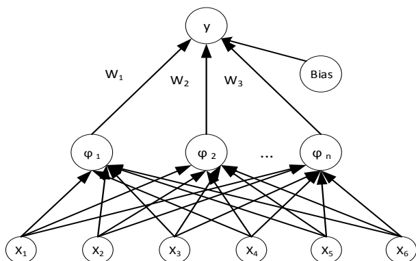
Gambar 1. Arsitektur Jaringan untuk prediksi Kecepatan Angin
