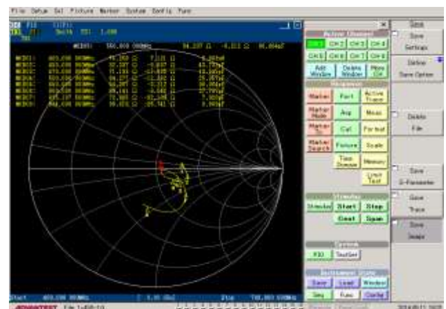
Gambar 5. Impedansi Hasil Pengukuran Prototipe Antena Mikrostrip DP-GP CSRR.
