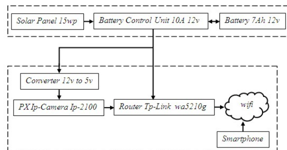
Gambar 1. Blok Diagram Sistem Kamera Pengamatan Bawah laut
