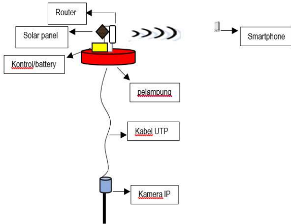
Gambar 2. Sistem kerja kamera bawah laut
