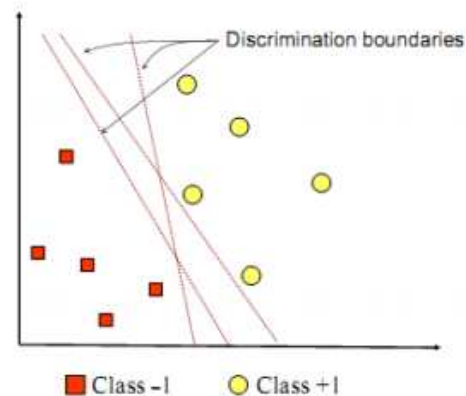
Gambar 2 Hyperplane terbentuk di antara kelas -1 dan +1
