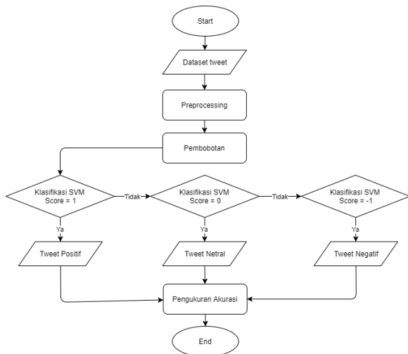
Gambar 4. Flowchart Klasifikasi SVM
