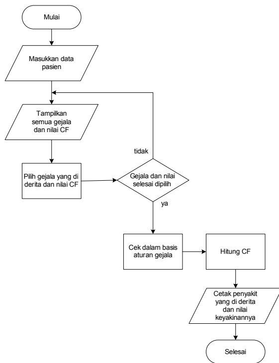
Gambar 2. Diagram alir konsultasi sistem pakar
