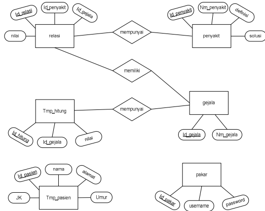
Gambar 5. ERD sistem pakar
