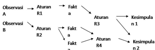
Gambar 1. Pelacakan Kedepan Forward Chaining .
