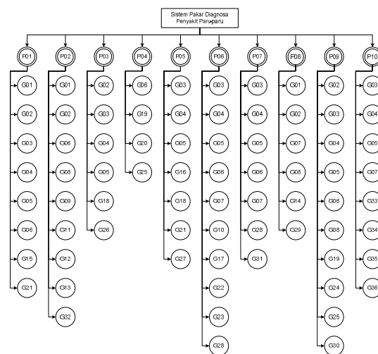
Gambar 6. Pohon keputusan.
