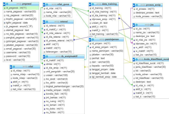
Gambar 2. Implementasi Database
