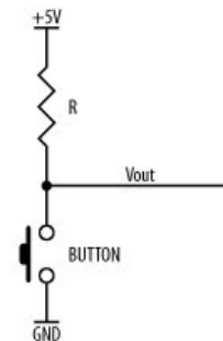
Gambar 7. Perancangan Rangkaian Push Button
