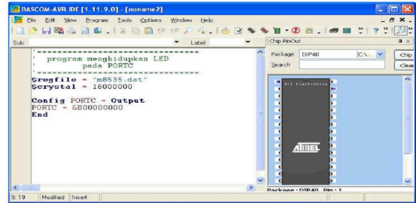
Gambar 4. Tampilan Bascom-AVR
