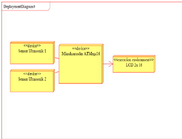
Gambar 8. Deployment diagram sistem penghitung jumlah pengunjung
