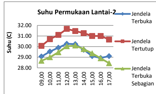
Gambar 11. Grafik suhu permukaan lantai 2
