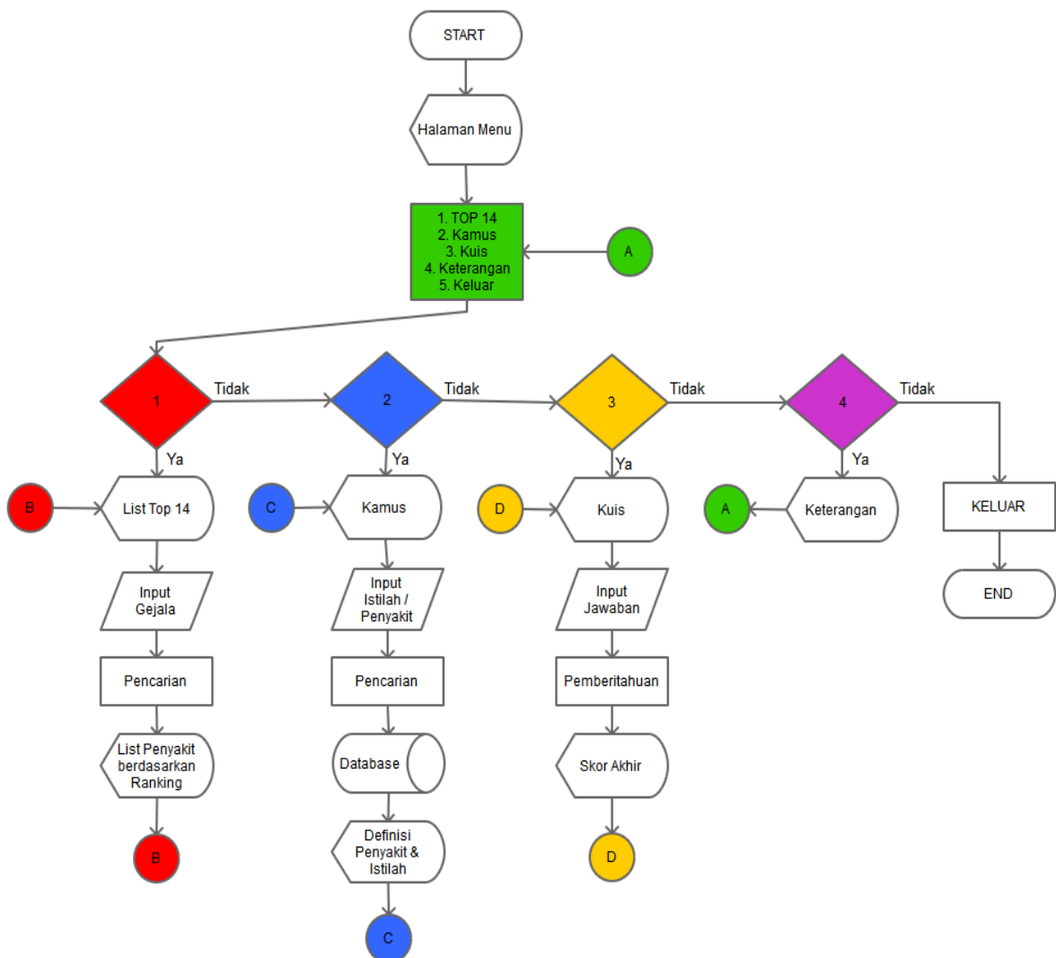
Gambar 2 Flowchart System secara umum
