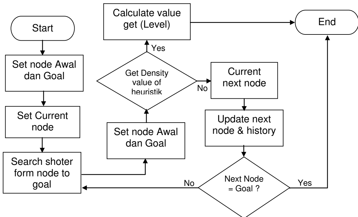
Gambar 1 Flowchat Alir Game dengan Algoritma A*
