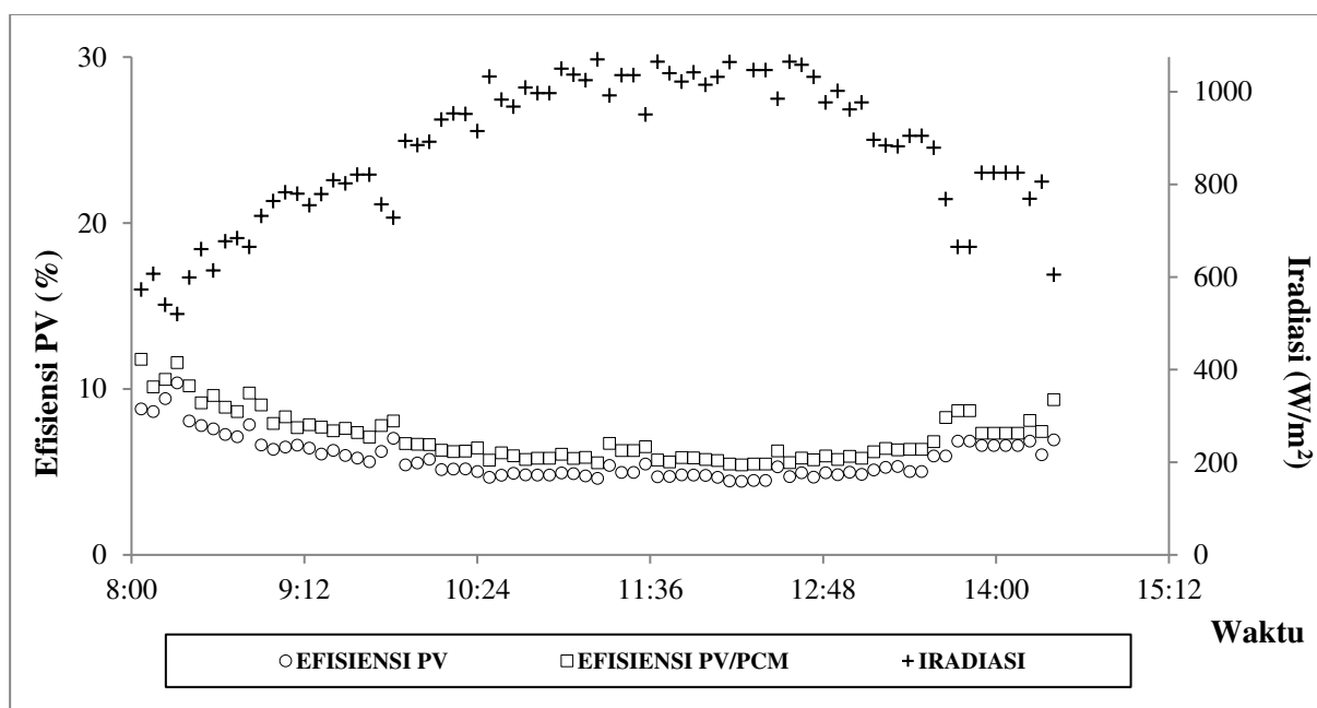
Gambar 8. Grafik efisiensi elektrik PV dan PV/PCM serta iradiasi matahari.
