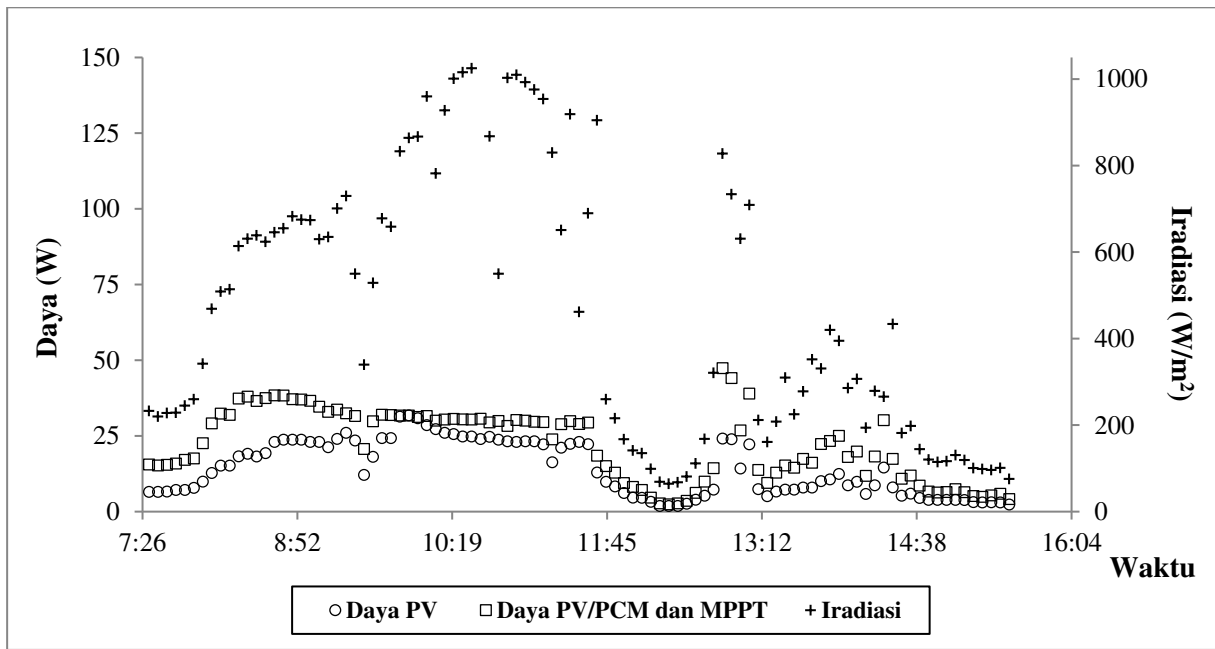
Gambar 15. Grafik daya PV dan PV/PCM & MPPT serta iradiasi matahari.
