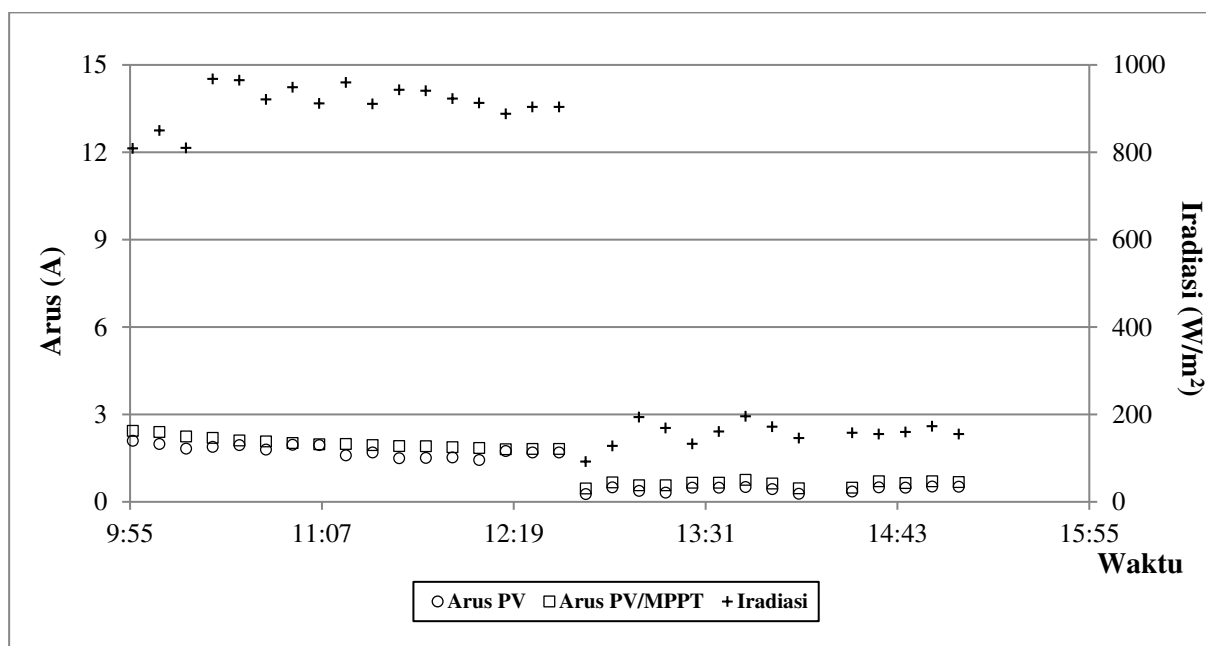
Gambar 10. Grafik arus PV dan PV/MPPT serta iradiasi matahari.
