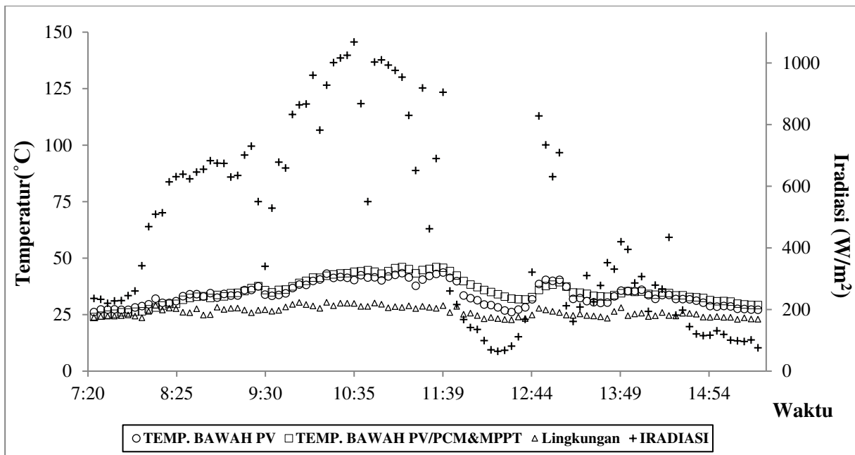
Gambar 14. Grafik temperature bawah PV dan PV/PCM & MPPT serta iradiasi matahari.
