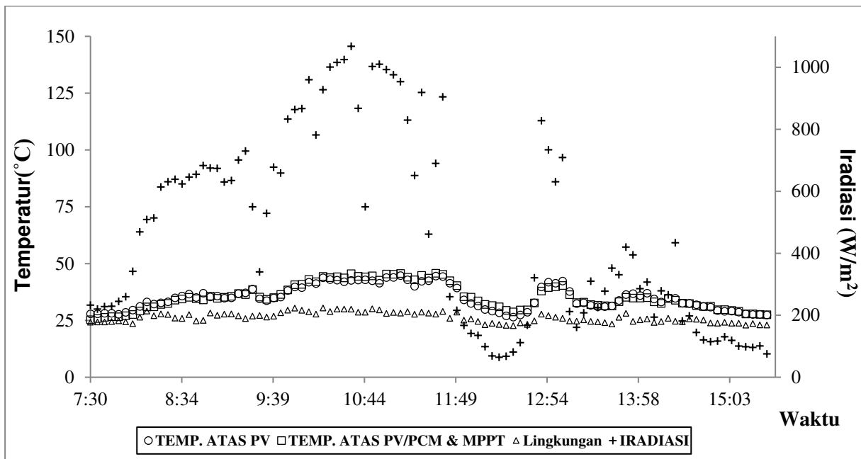
Gambar 13. Grafik temperature atas PV dan PV/PCM & MPPT serta iradiasi matahari.
