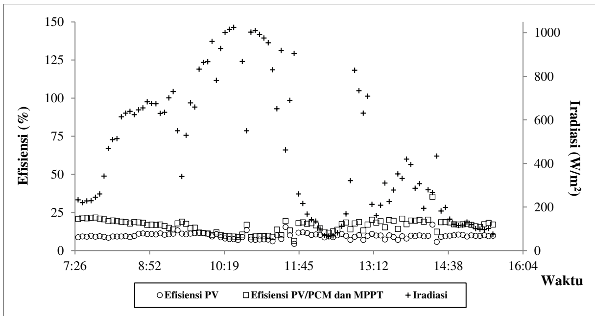
Gambar 16. Grafik efisiensi PV dan PV/PCM & MPPT serta iradiasi matahari.
