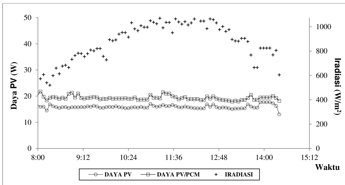
Gambar 7. Grafik daya PV dan PV/PCM serta iradiasi matahari.
