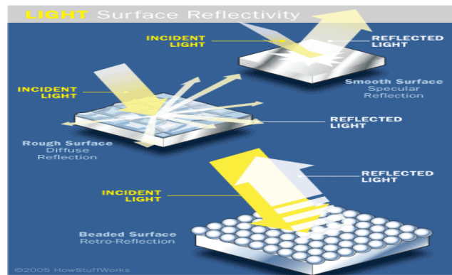
Fig 4 :-Retro-reflective material
