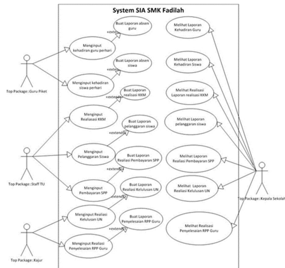
Gambar 4 Use Case yang berjalan
