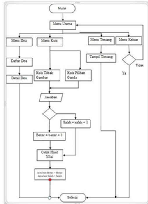
Gambar 1. Flowchart Aplikasi Doa Harian Anak
