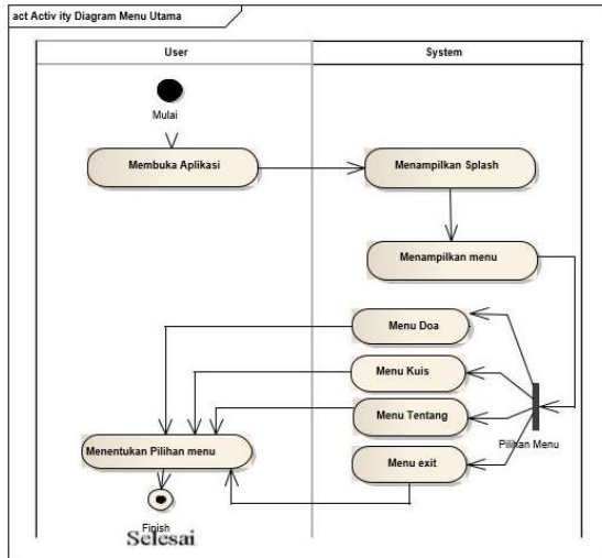
Gambar 3. Activity Diagram Menu Utama Aplikasi
