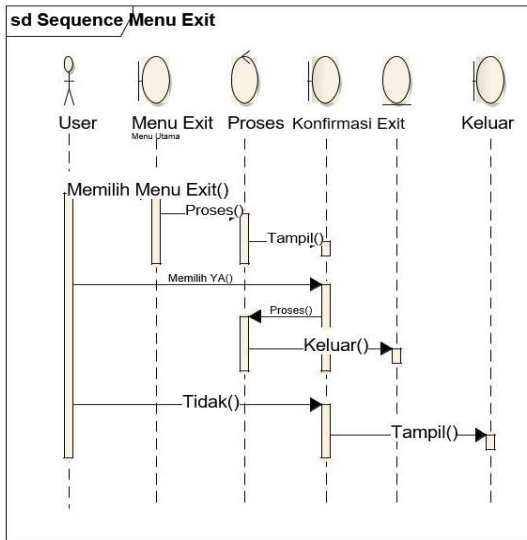
Gambar 11. Sequence Diagram Menu Keluar
