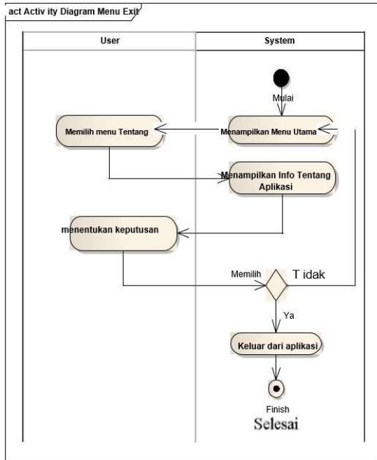
Gambar 7. Activity Diagram Menu Keluar Aplikasi
