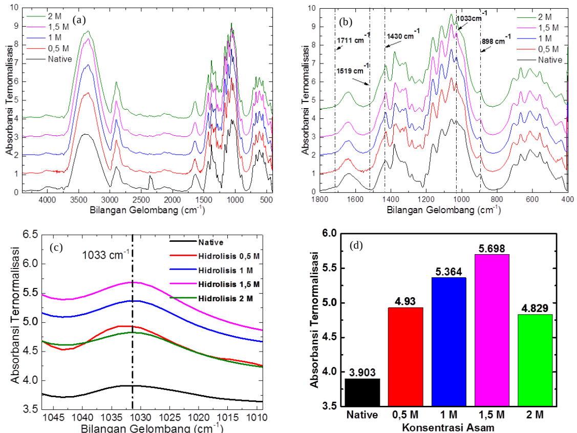
Gambar 4. (a). Spektrum FT-IR kapas limbah dan hasil ekstraksi pada berbagai konsentrasi asam, (b). Segmen spektrum wilayah fingerprint pada bilangan gelombang 1800 cm -1 hingga 400 cm -1 , (c). Segmen spektrum FT-IR pada bilangan gelombang 1050 cm -1 hingga 1000 cm -1 dan (d). Kecenderungan nilai absorbansi pada masing masing hasil hidrolisis pada bilangan gelombang 1033cm -1 .
